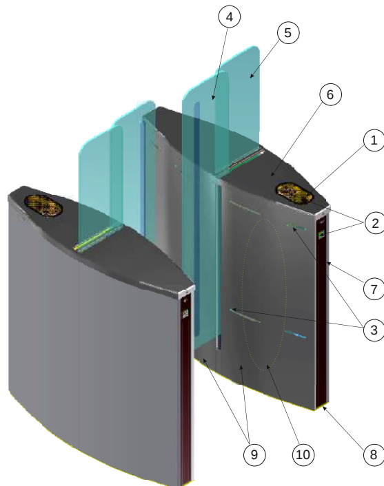
Рис. 4 – Конструкція турнікета «JETPAN-BM-1» однопрохідного ТЗ.KCD.XK
