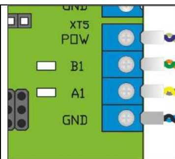
Рис.21 – Підключення кабелю зв'язку з пультом керування до клем АЮІА.206.21.20.00
