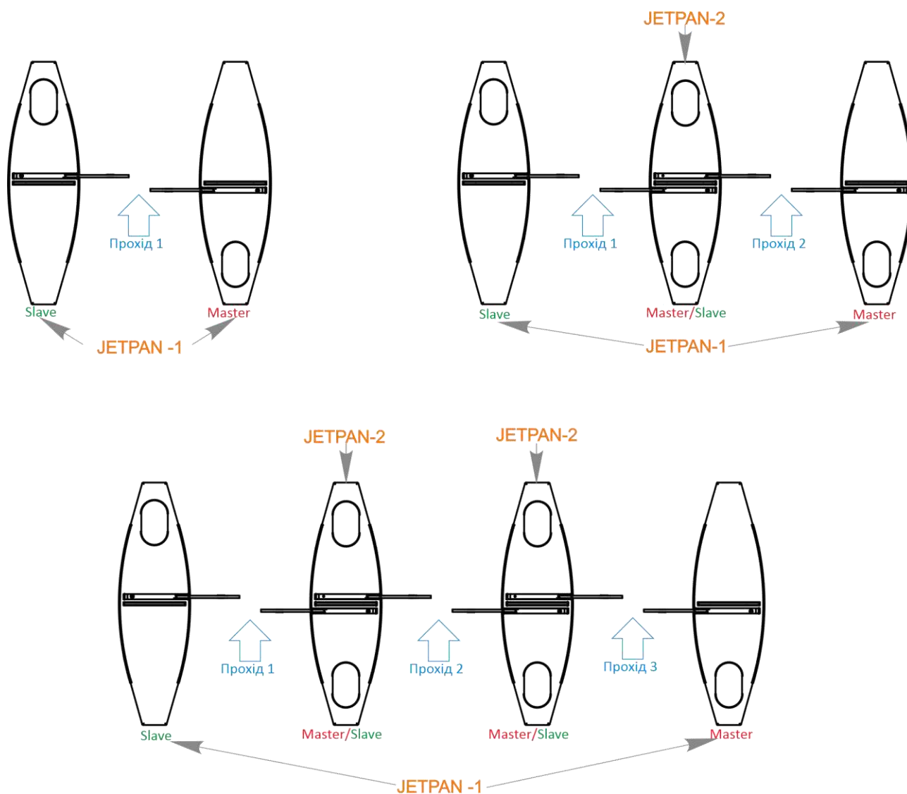
Рис.14– Варіанти розміщення турнікетів типу «JetPan-BM»
