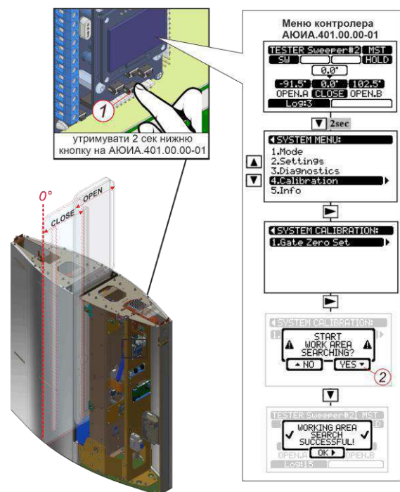
Рис.24 – Встановлення нульового положення стулки за допомогою кнопки «zero»
